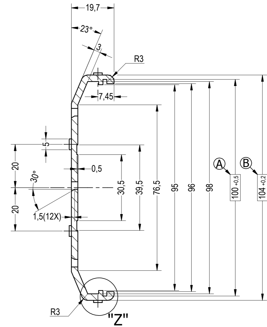
Corte A-A esc. (1:1)
