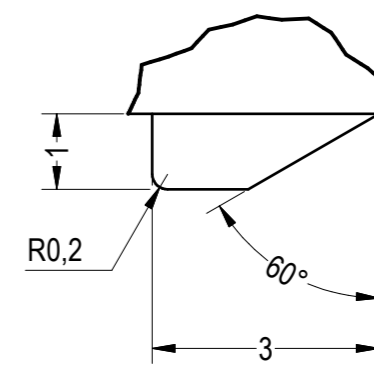
Det."X" esc. (10:1)
