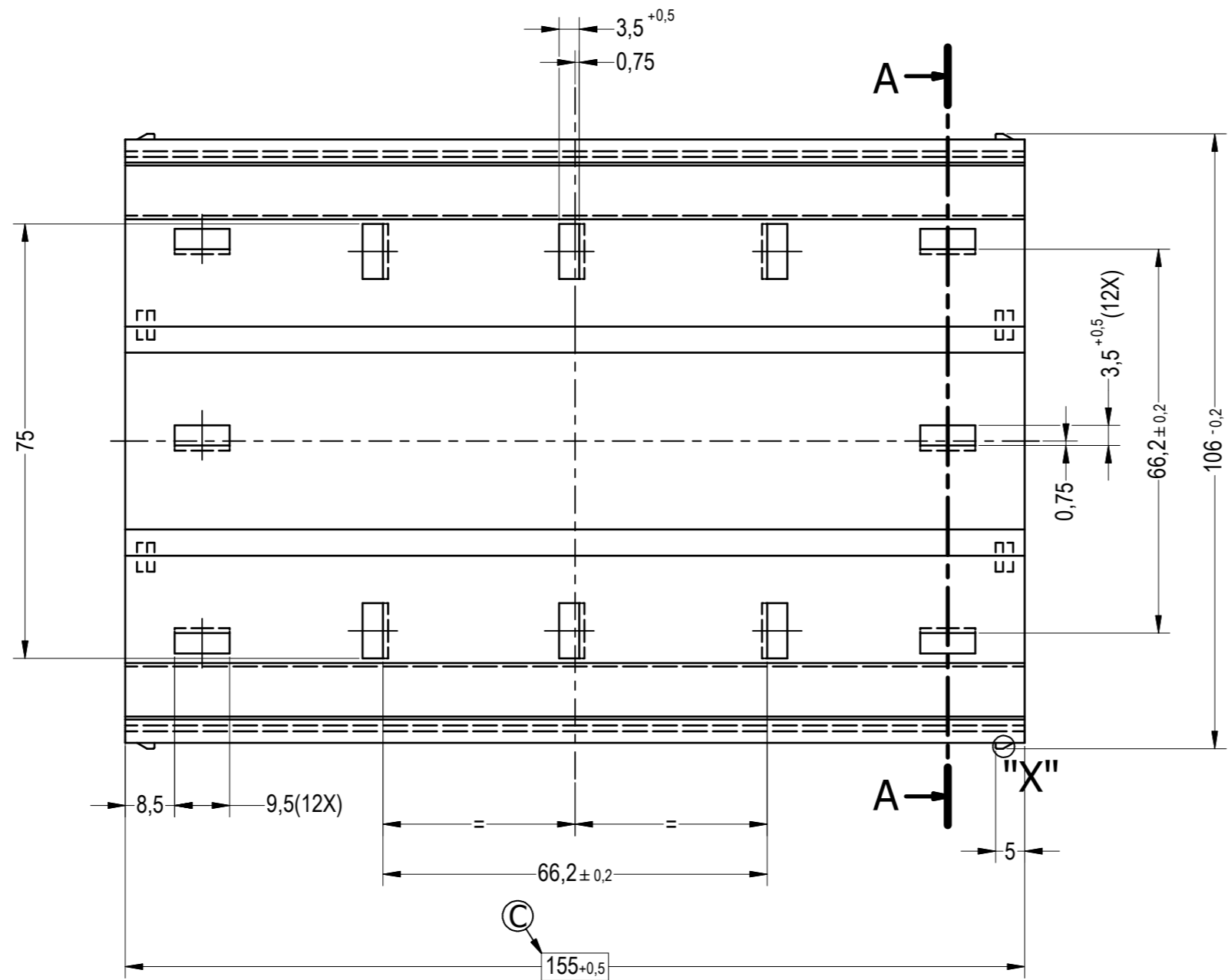
PEÇA COM 155MM DE COMPRIMENTO CÓDIGOS VIDE TABELA
