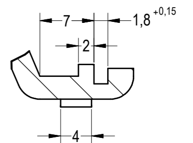
Det."Z" esc. (2:1)
