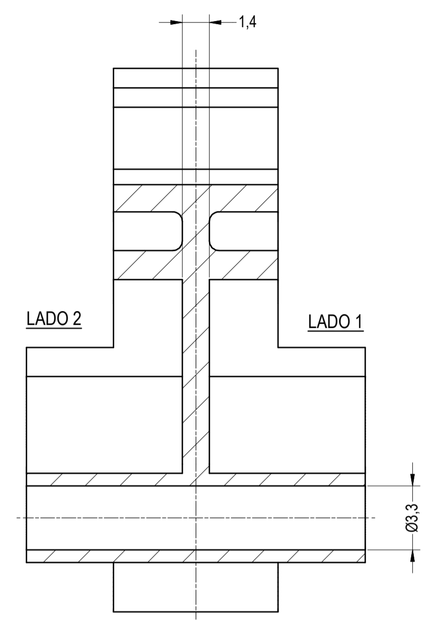
CORTE B-B
