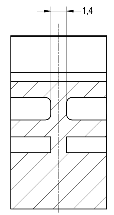
CORTE D-D
