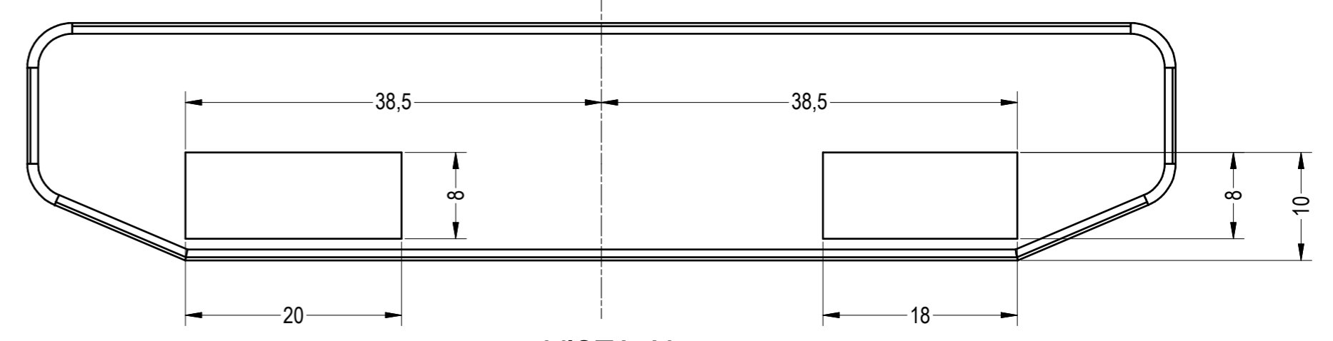
VISTA X
