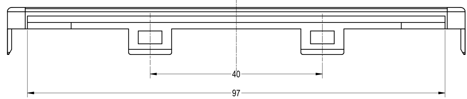
CORTE B-B
