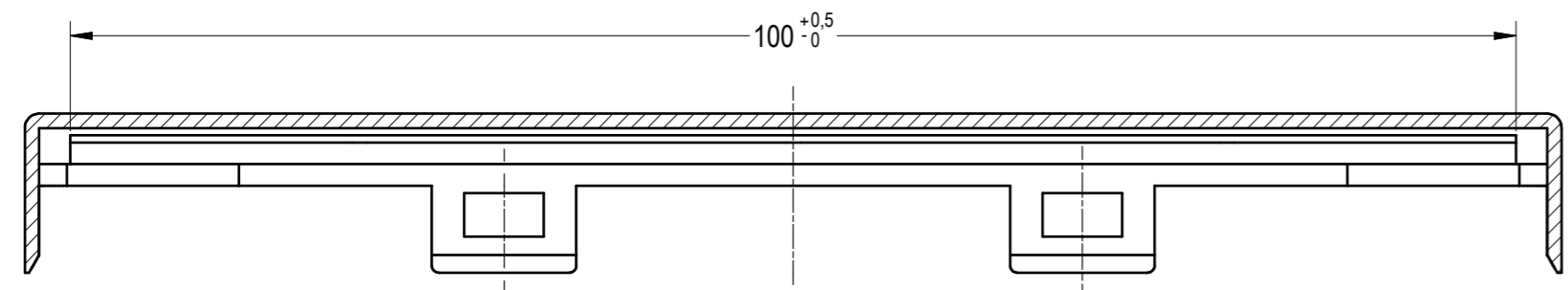
CORTE B-B
